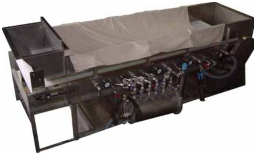
ブロック別の温度管理
